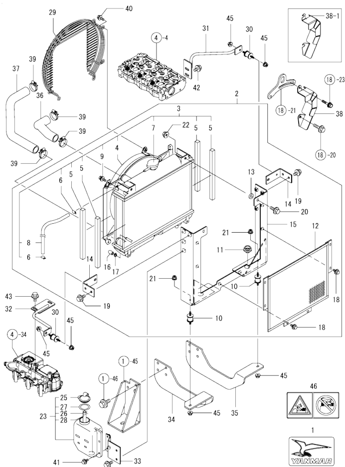
Fig.11. RADIATOR
